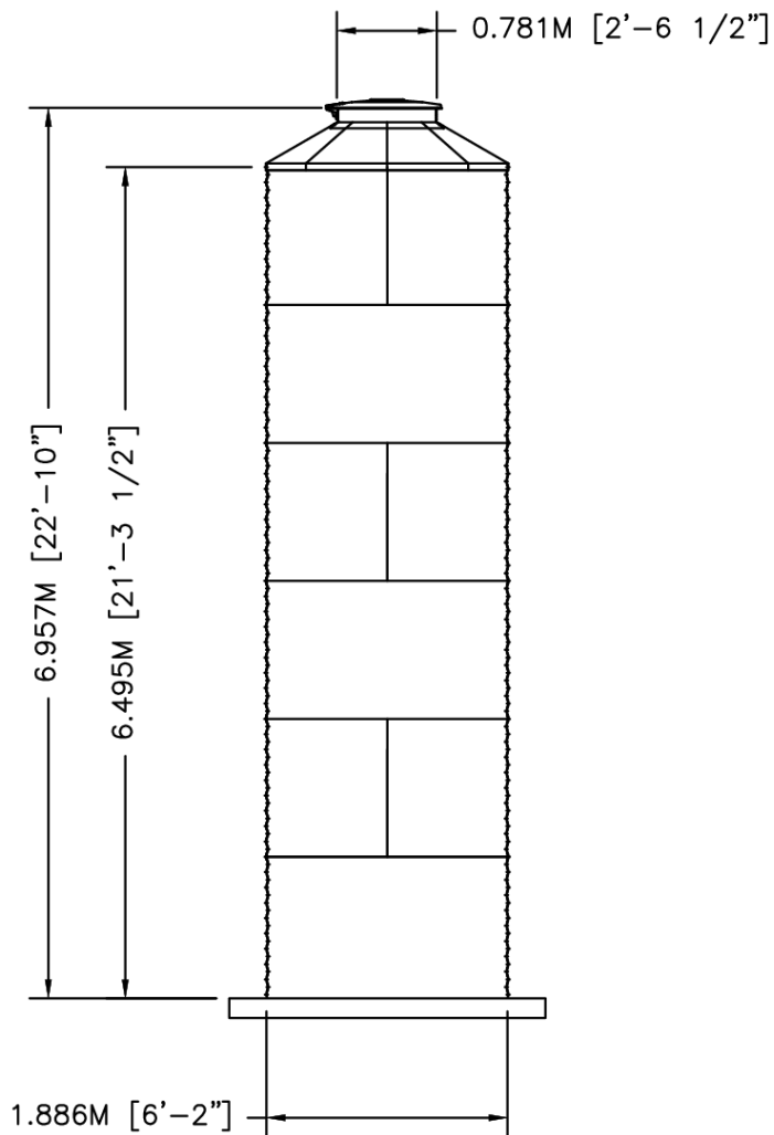
ELEVATION
